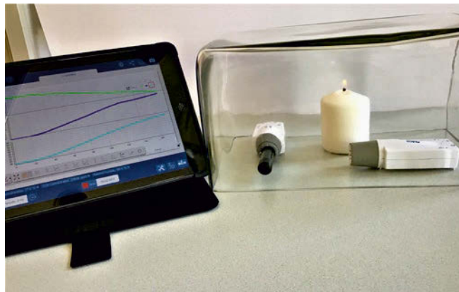
▲ Abb. 2 Aufbau und Durchführung des Experiments
