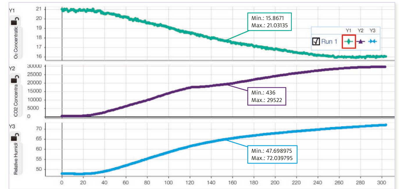
▲ Abb. 3 Darstellung der Konzentrationsänderungen im Reaktionsverlauf
