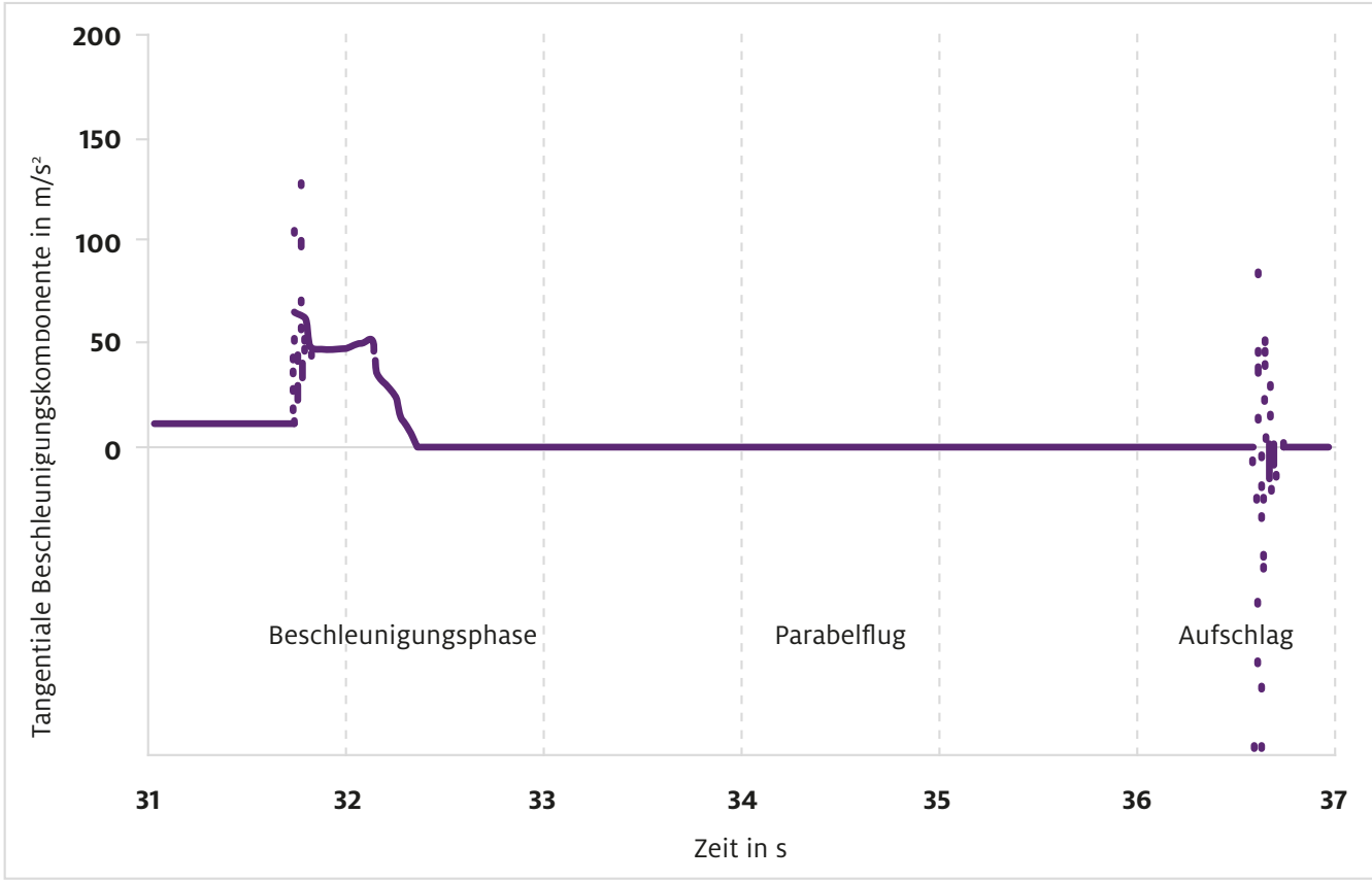
▲ Abb. 2 Digitale Messung der tangentialen Beschleunigungskomponente von einem Smartphone in einer Druckwasserrakete (Messung: Mayer, Söder, Mauch)
