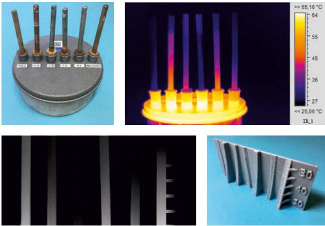
◀ Abb. 2 Wärmebilder als Beispiel für Multicodierung und Multimodalität
